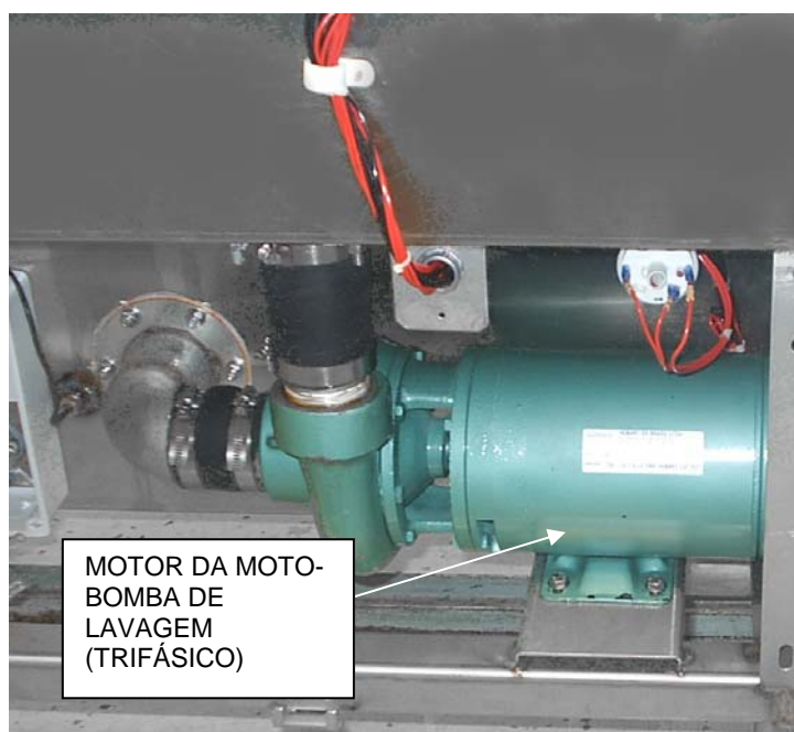
Fig. 7 (Ref.: Lavadora CA112B Esquerda p/ Direita)
